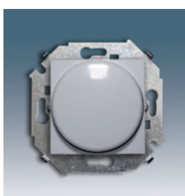
1591311 -030 -031 -032 -033 -034 -036 Светорегулятор поворотной-нажимной, электронный, проходной, 20-500 Вт 1591790 -030 -031 -032 -033 -034 -036 Светорегулятор поворотной-нажимной, электронный, проходной, 20-500 Вт Лампы накаливания, галогенные лампы, галогенные с электрон./электромагнит. трансформатором 230В/12В
